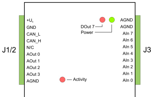
Abbildung 4: Anschlüsse der Grundplatte Analog 1
