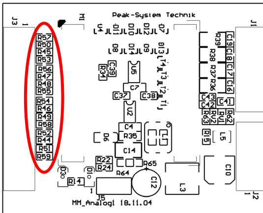
Abbildung 3: Position der Widerstände zur Messbereichserweiterung
