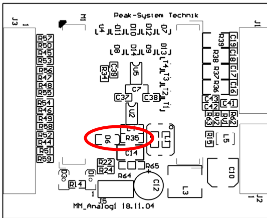
Abbildung 2: Positionen D6 und R35
