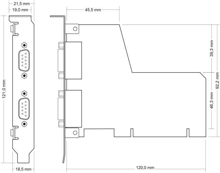
PCAN-PCI Zweikanal
