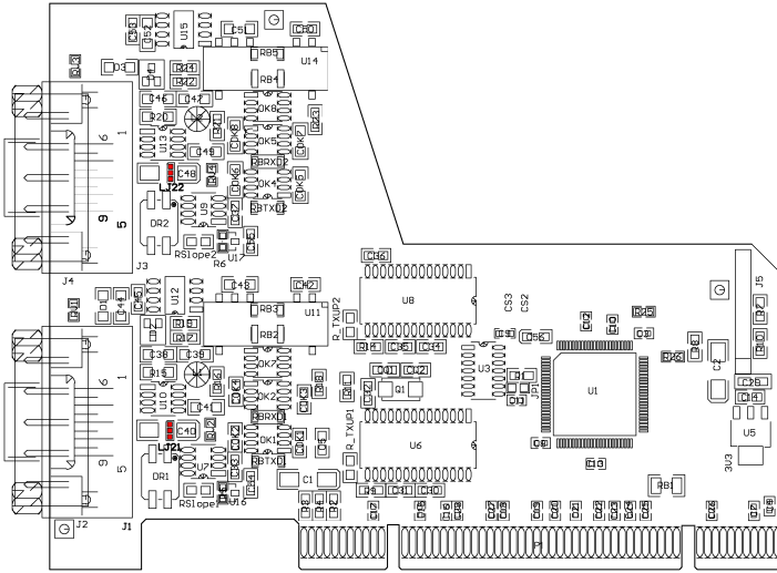
Position der Lötfelder für die 5-V-Versorgung am CAN-Anschluss
